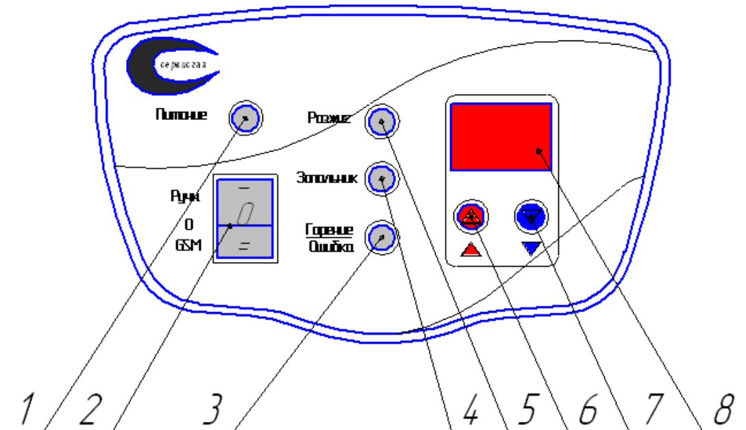
Рис.4 Блок управления
