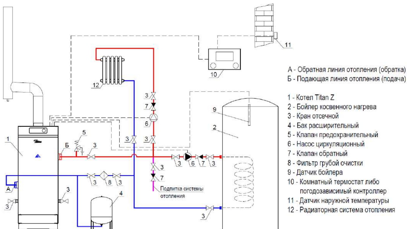
Рисунок 4. Вариант схемы подключения котла с контуром отопления и бойлером ГВС
