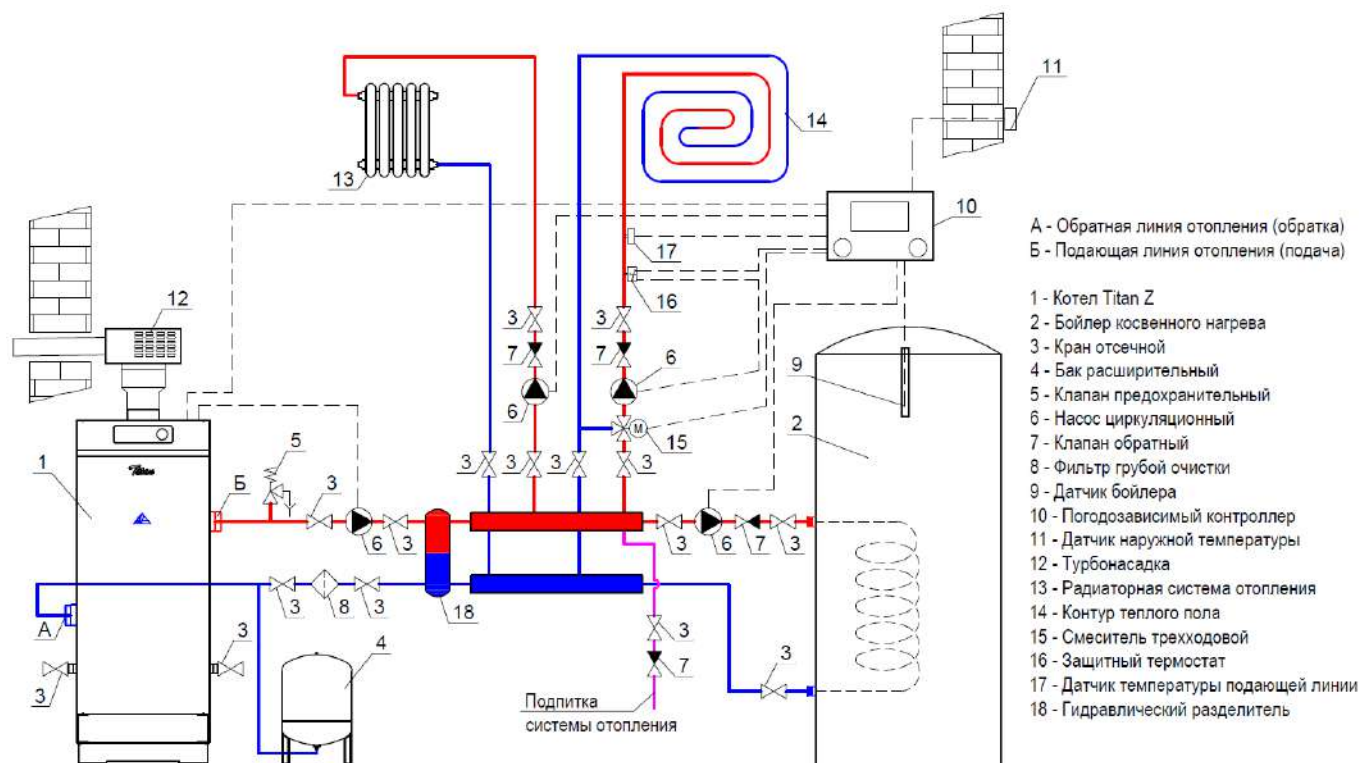
Рисунок 6. Вариант подключения котла в схеме с гидравлическим разделителем (стрелкой)
