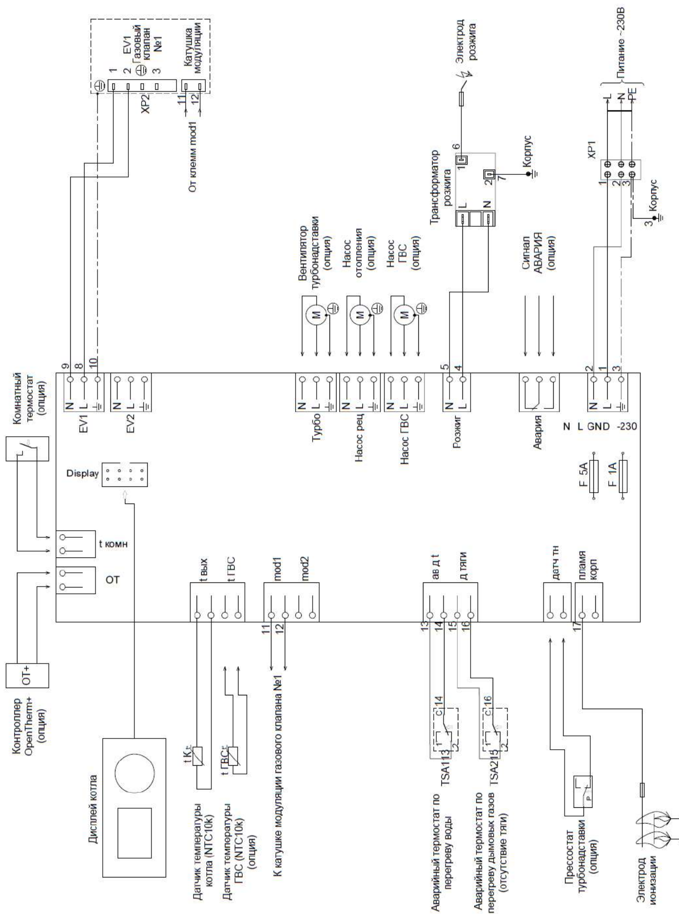
Рисунок 7. Электрическая схема котлов TITAN Z30M; Z40M; Z50M; Z60M; Z65M
