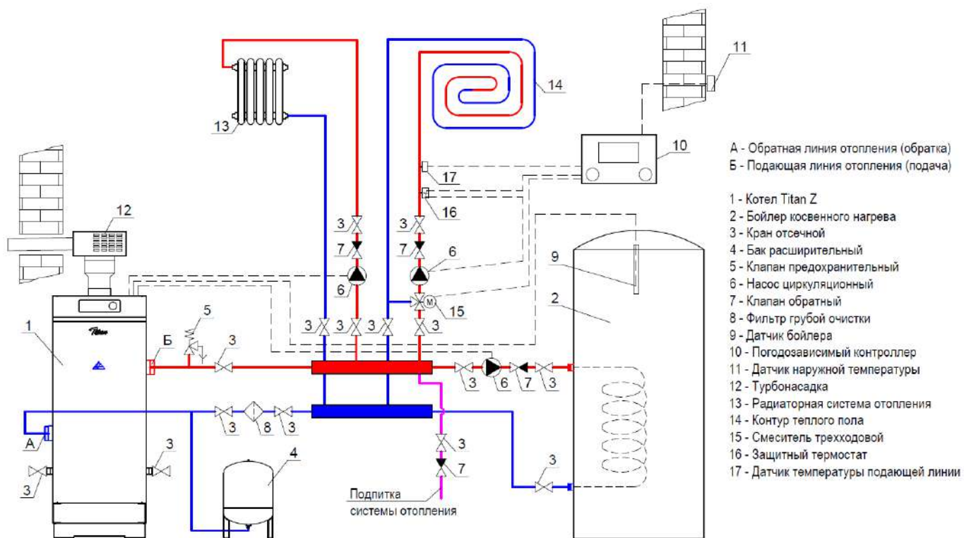
Рисунок 5. Вариант подключения котла в схеме с коллектором
