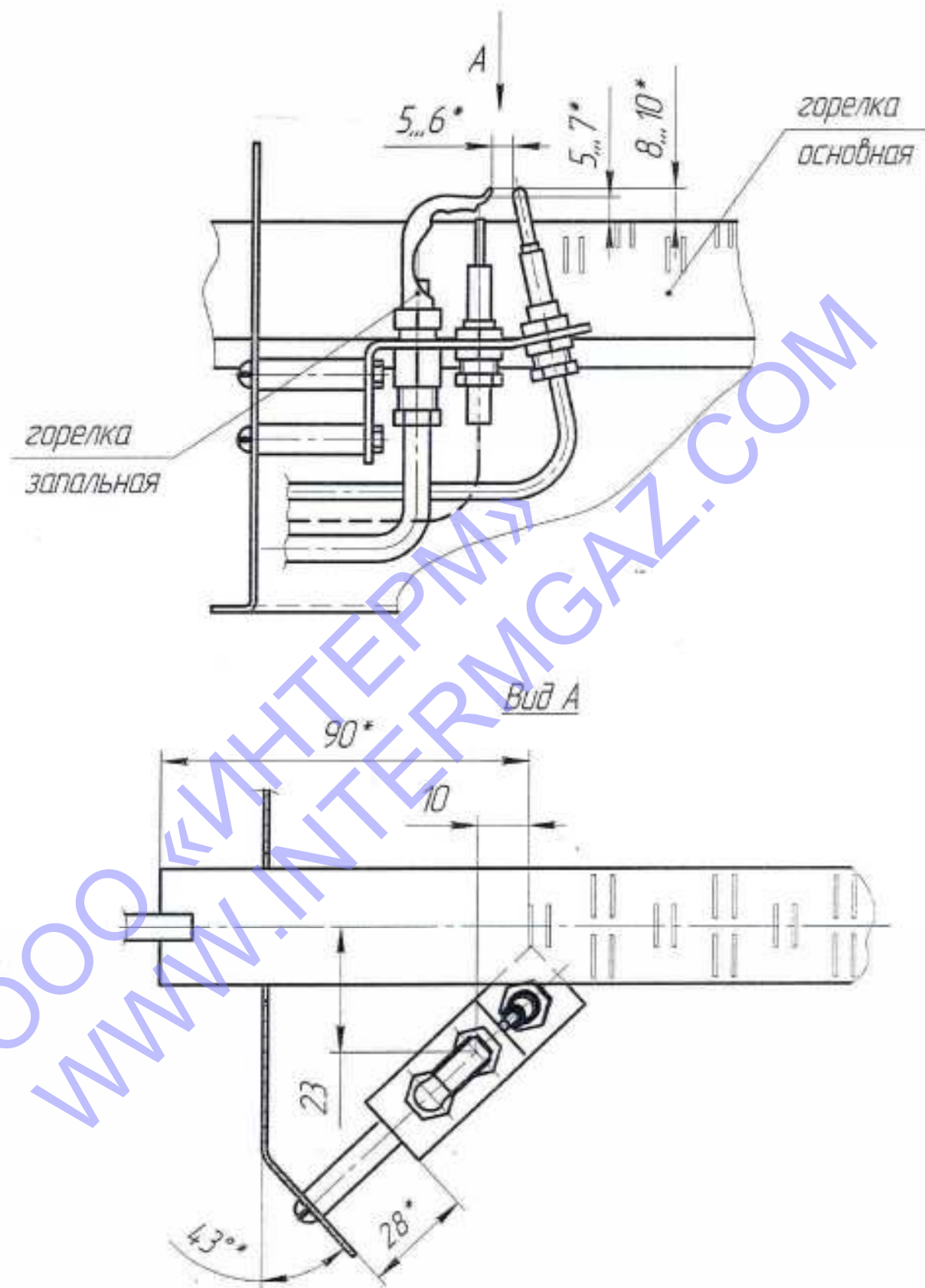
Рис. 4 А . Схема расположения горелки запальной относительно основной.
