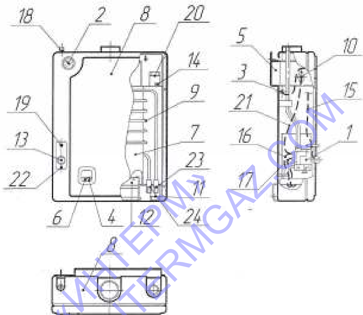
Рис. 1 Конструкция котла
