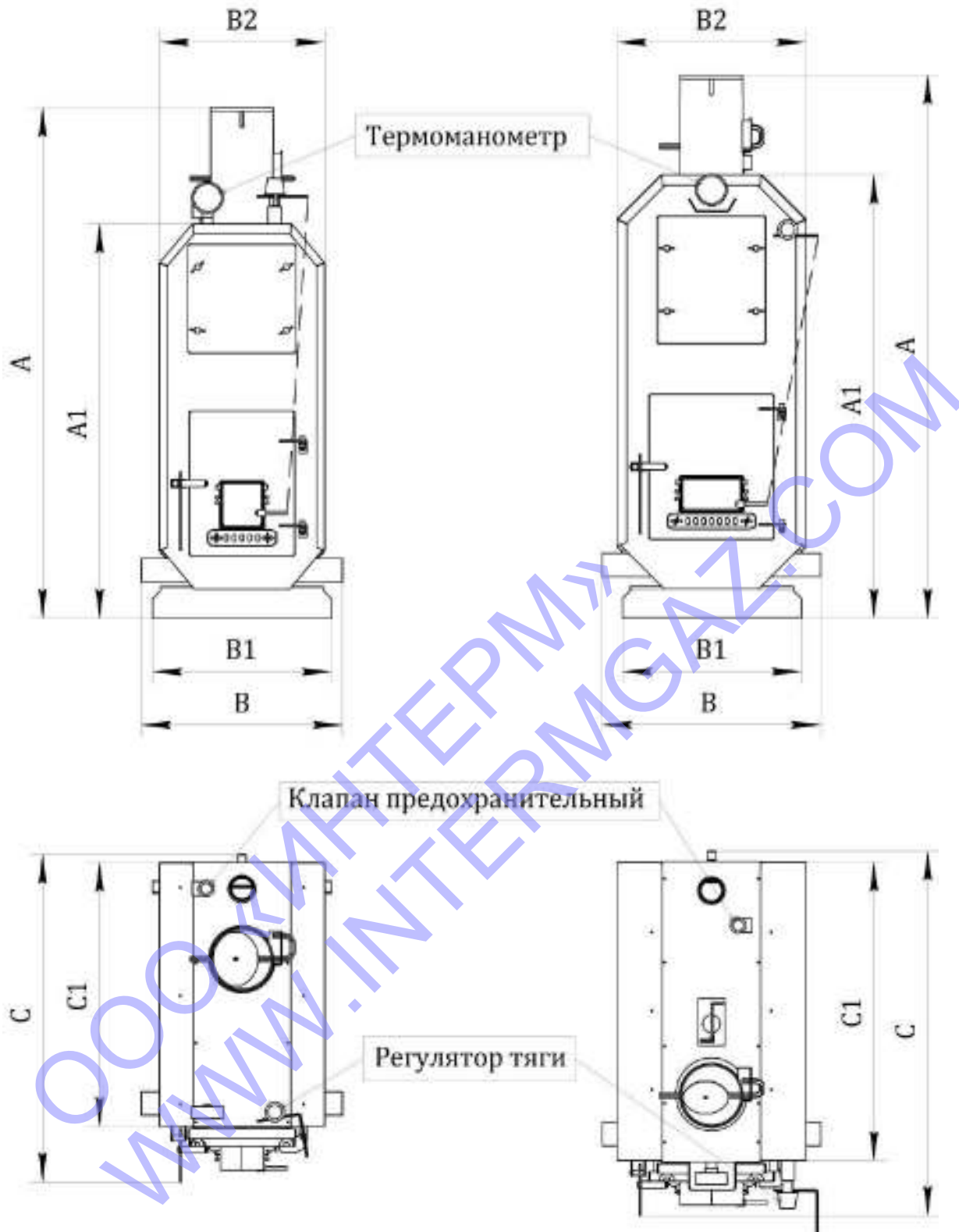
Рисунок 4 - Общий вид и оснащение котла с вертикальной дымовой трубой
