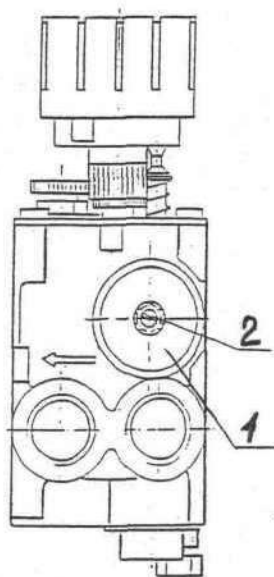
Рис. 3. Элементы регулировки газового клапана.
