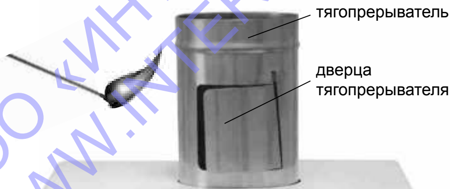
Рисунок 7. Тягопрерыватель
