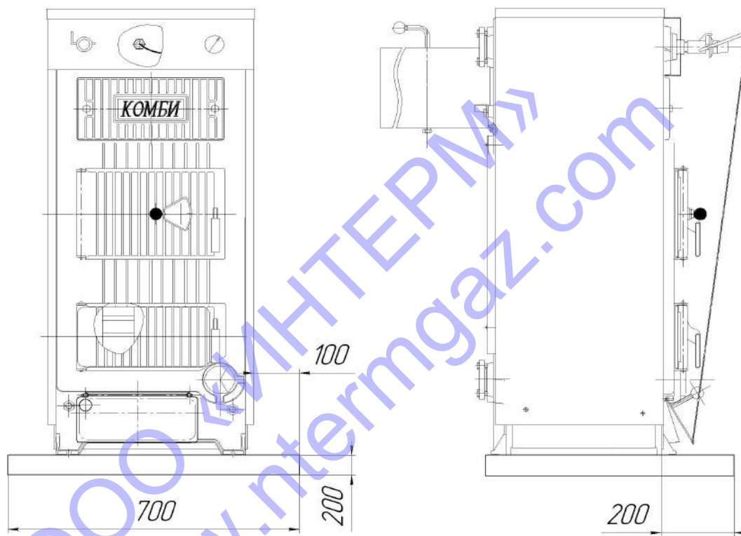
Рис. 5.1 Размеры цоколя
