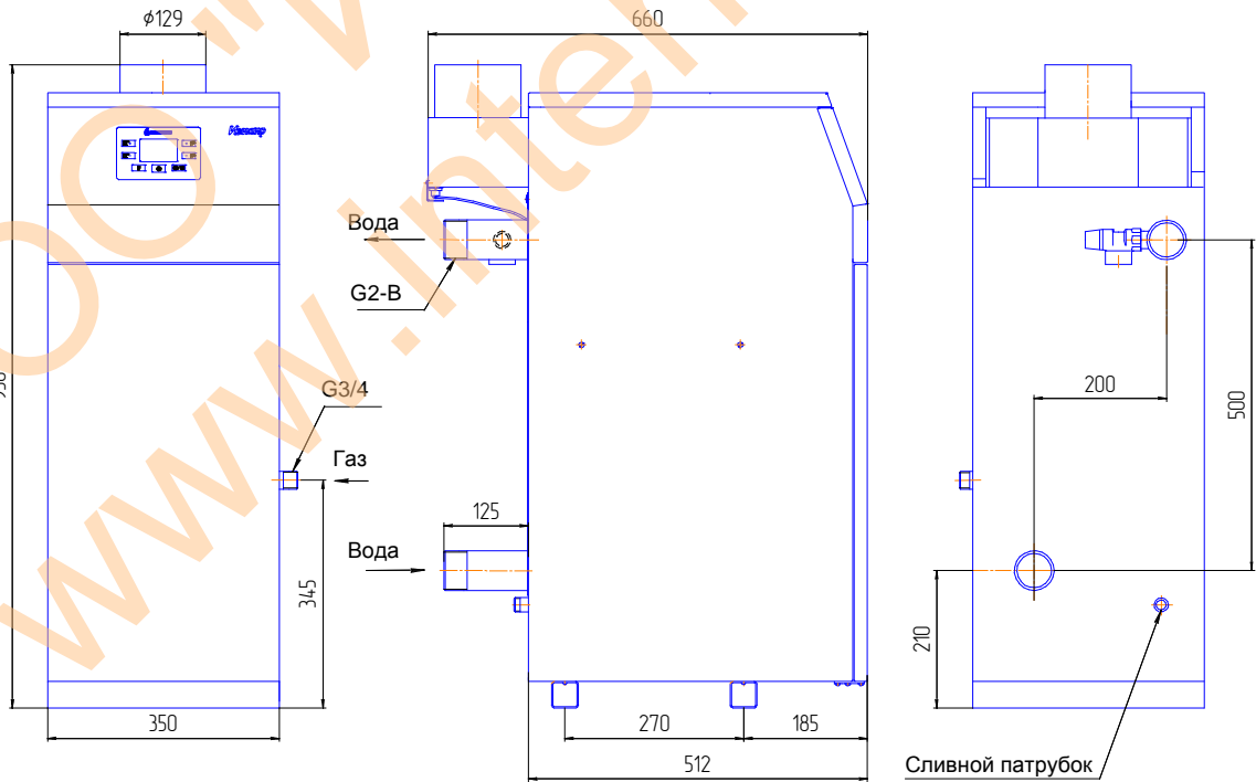
Рисунок 3. Габаритные и присоединительные размеры котлов.
