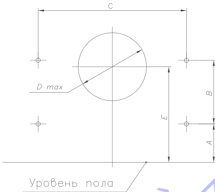
Рисунок 5. Схема расположения отверстий под крепления аппарата (котла)
