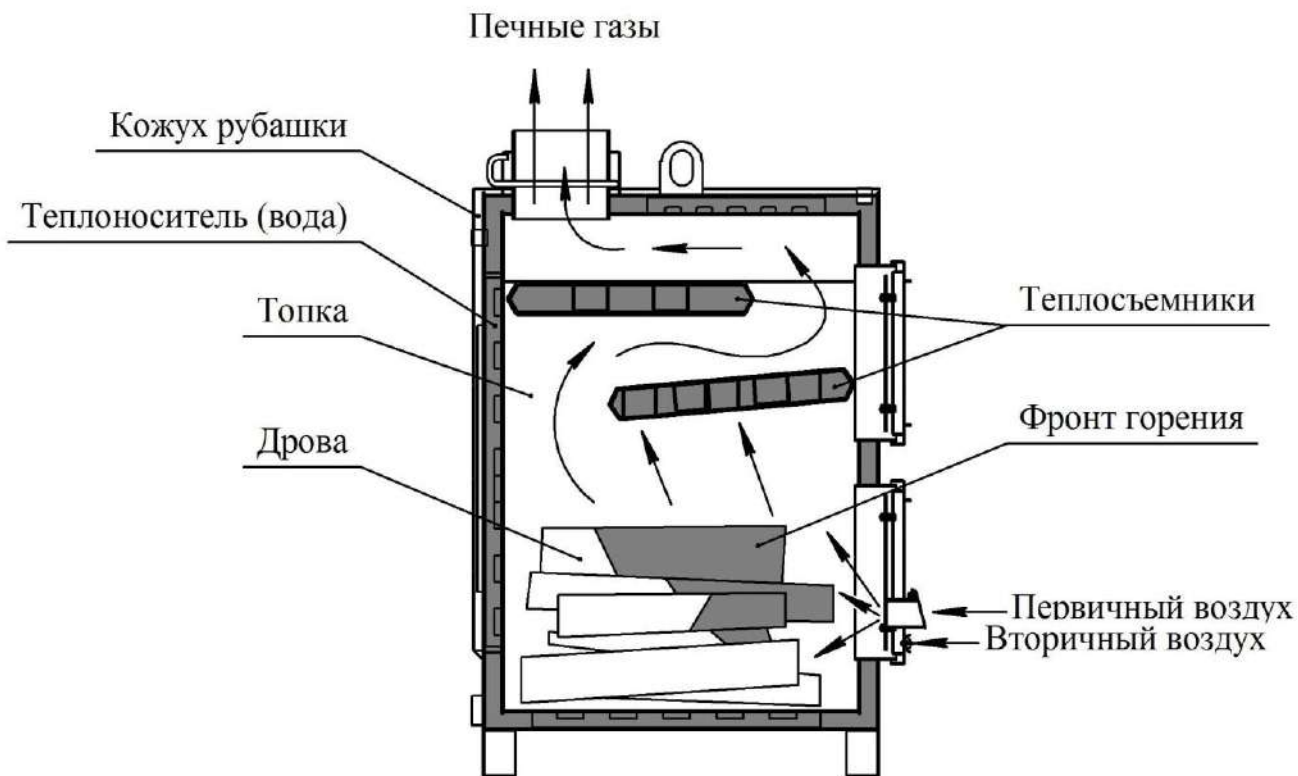
Рисунок 1 - Схема КОД-50
