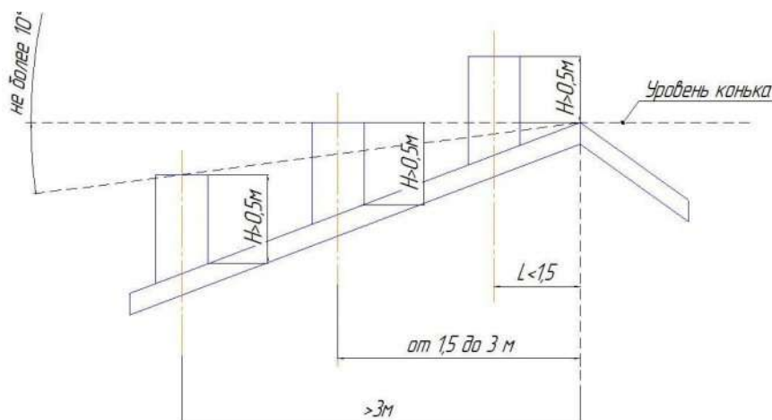
Рисунок 11 – Варианты расположения трубы на скате
