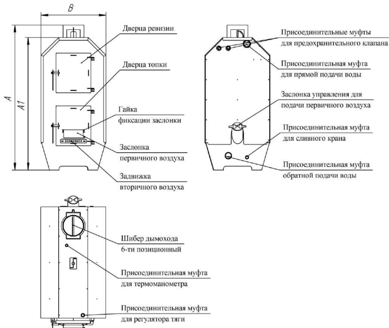
Рисунок 4 – Общий вид и оснащение котла
